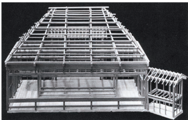
農村舞台軸組模型
